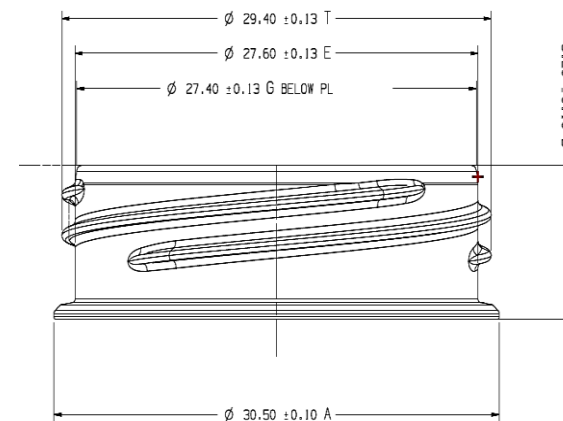
Rosca 29/25
